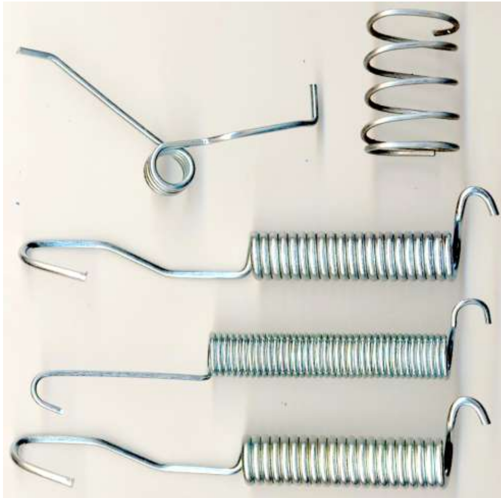
CODIGO: 6056 RAM VAN WAGON TRADESMAN IZQUIERDO 91 – 97
