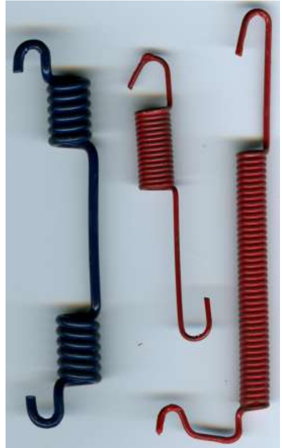
CODIGO: 6005 CHEVY – MONZA
