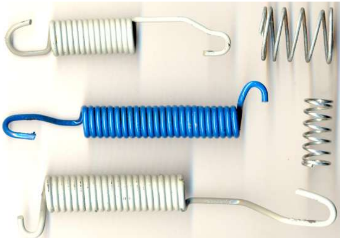
CODIGO: 6061 CHEVROLET MICRO C – 30 RT 90 – 01
