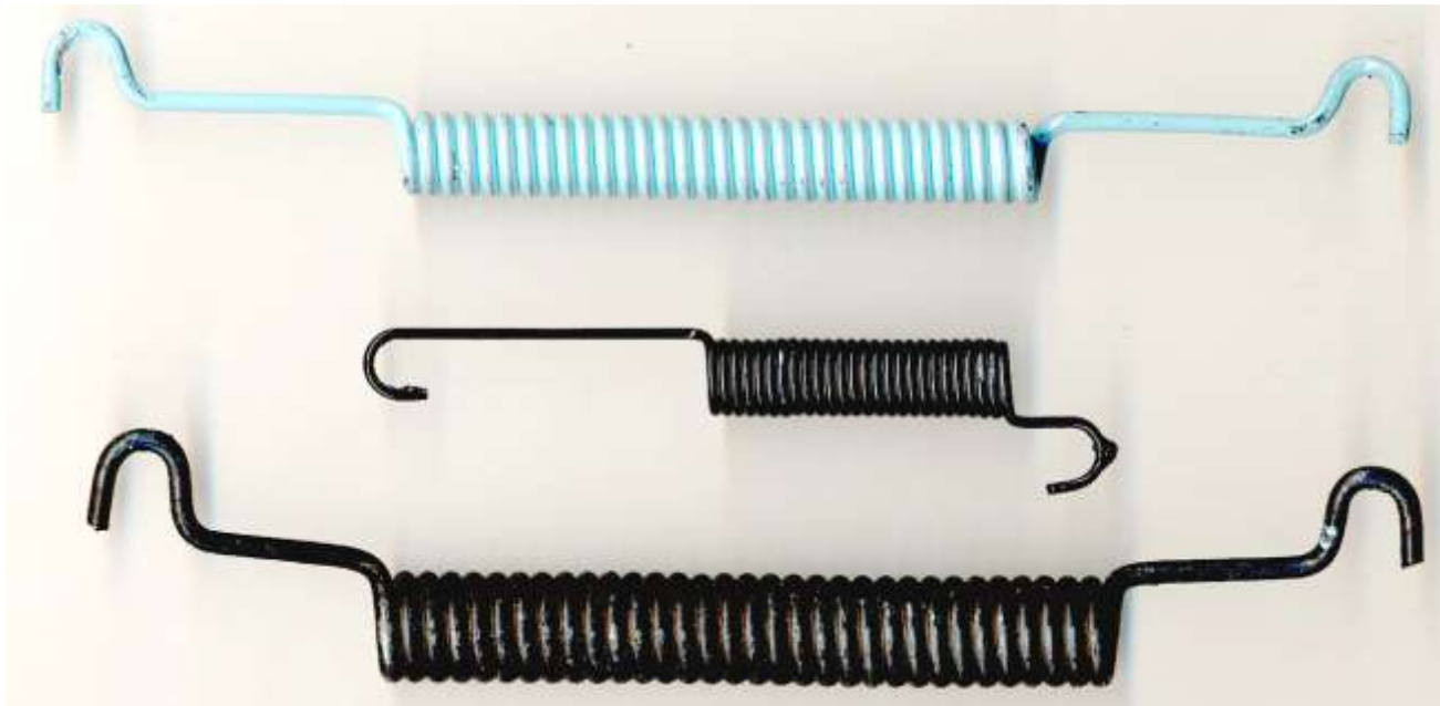
CODIGO: 6049 DATSUN PICK UP AMERICANA RT
