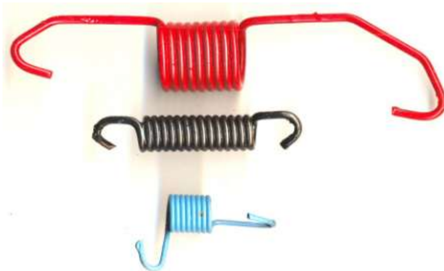
CODIGO: 6073 TOYOTA COROLLA 83 – 88
