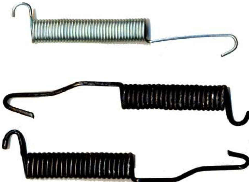
CODIGO: 6055 CHRYSLER – VOYAGER 91 – 95, DAKOTA 91 – 99
